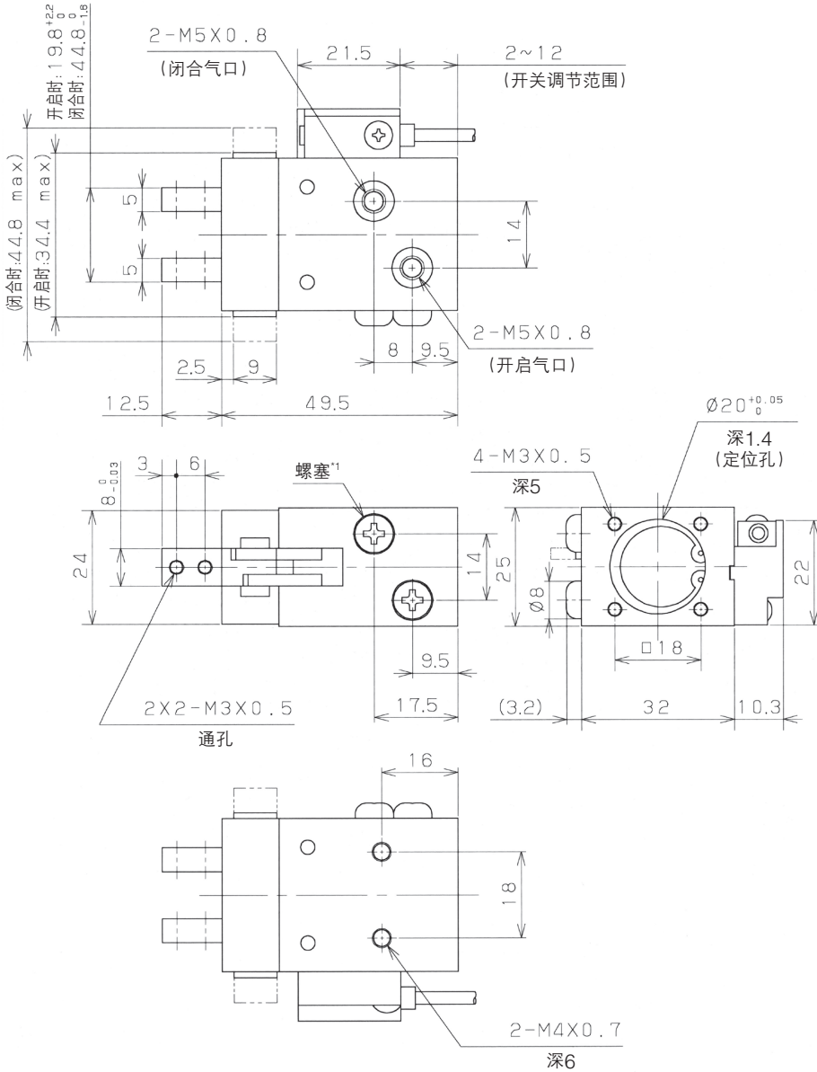
外形尺寸图 CKHL-16
