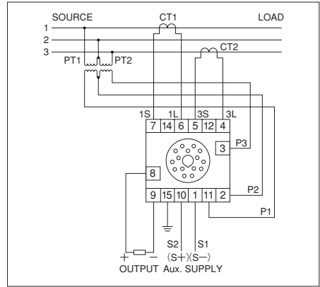
RHP-□3 三相3線
