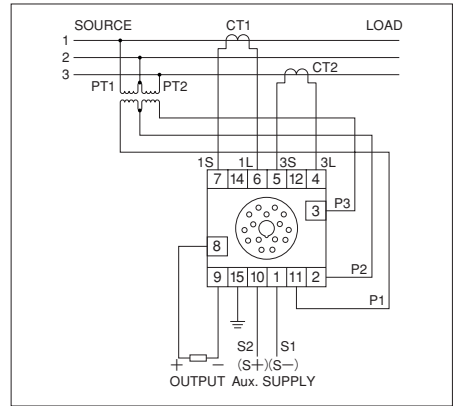
RHP-□2 単相3線
